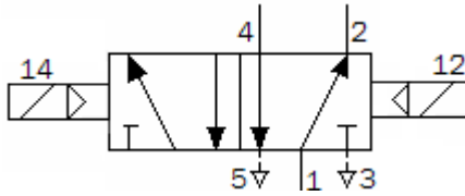
Electroválvula 5/2, biestable con servopilotaje
