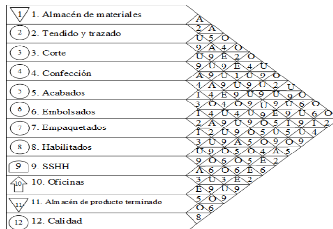
Gráfico 2. Diagrama de relaciones actual
