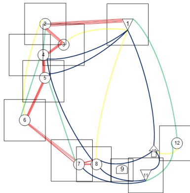
Gráfico 6. Diagrama de relaciones por bloques.
