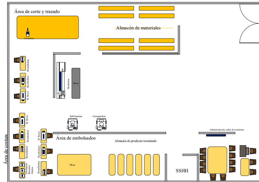
Gráfico 11. Disposición de equipos de trabajo
