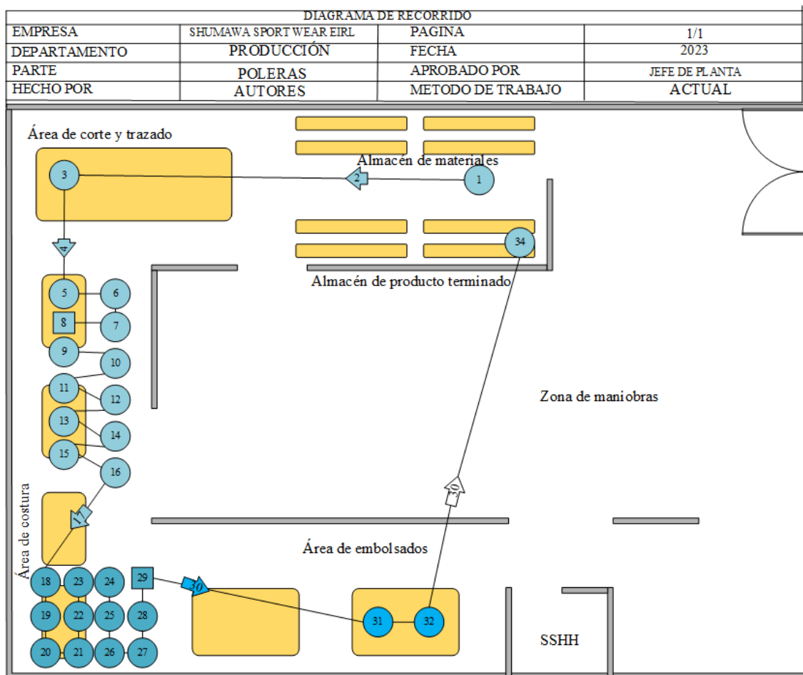
Gráfico 4. Diagrama de recorrido actual
