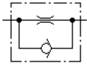
Válvula reguladora de caudal unidireccional con regulación fija
