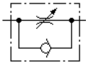
Válvula reguladora de caudal unidireccional con regulación variable
