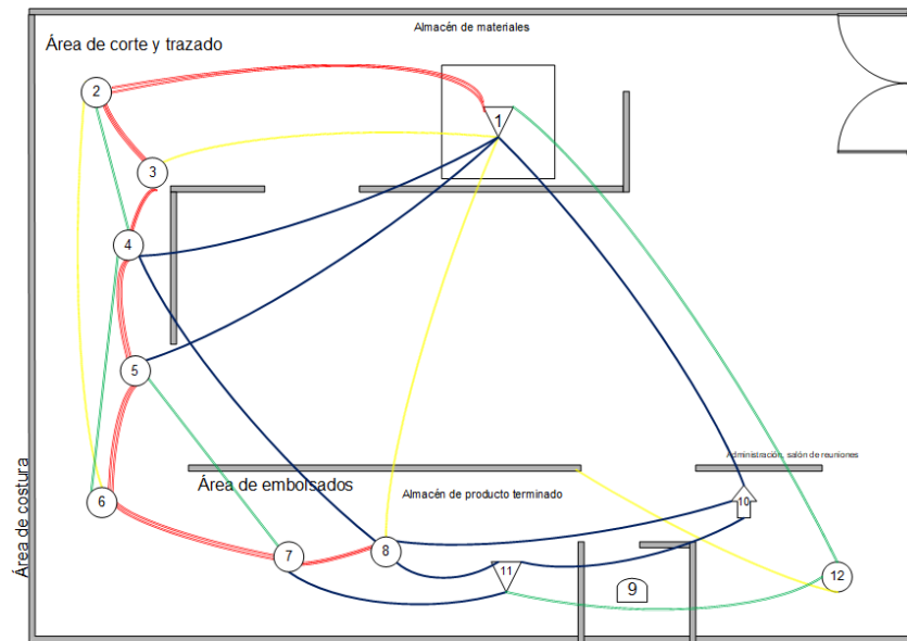
Gráfico 7. Diagrama de recorrido donde muestras las relaciones de cada zona.
