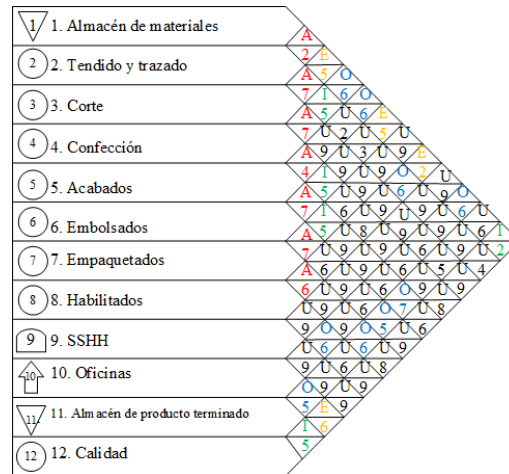
Gráfico 5. Diagrama de relaciones propuesto
