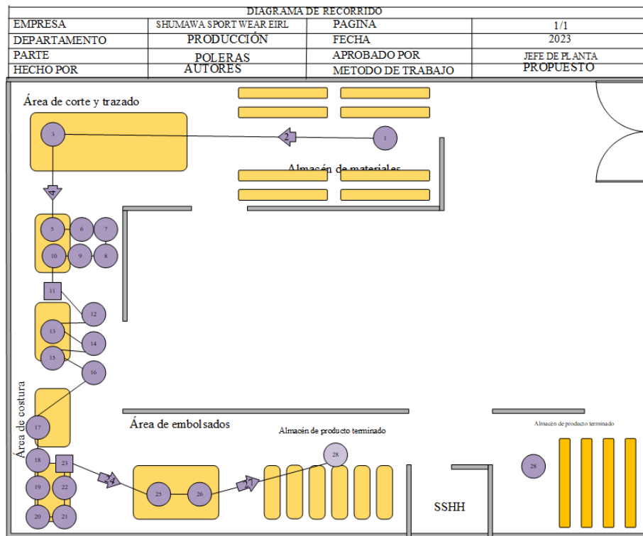
Gráfico 10. Propuesta de diagrama de recorrido propuesto
