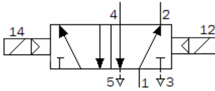
Electroválvula 5/2, biestable con servopilotaje
