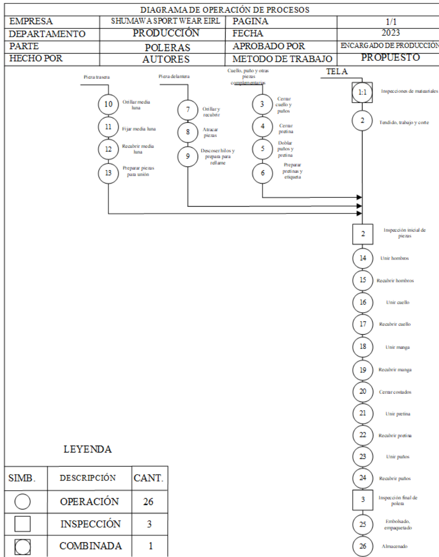
Gráfico 8. Propuesta de diagrama de operaciones del proceso de elaboración de poleras.
