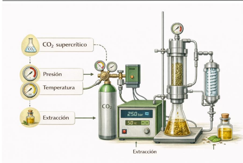
Figura 6. Representación esquemática de la extracción de compuestos fenólicos mediante \text{CO}_2 supercrítico
