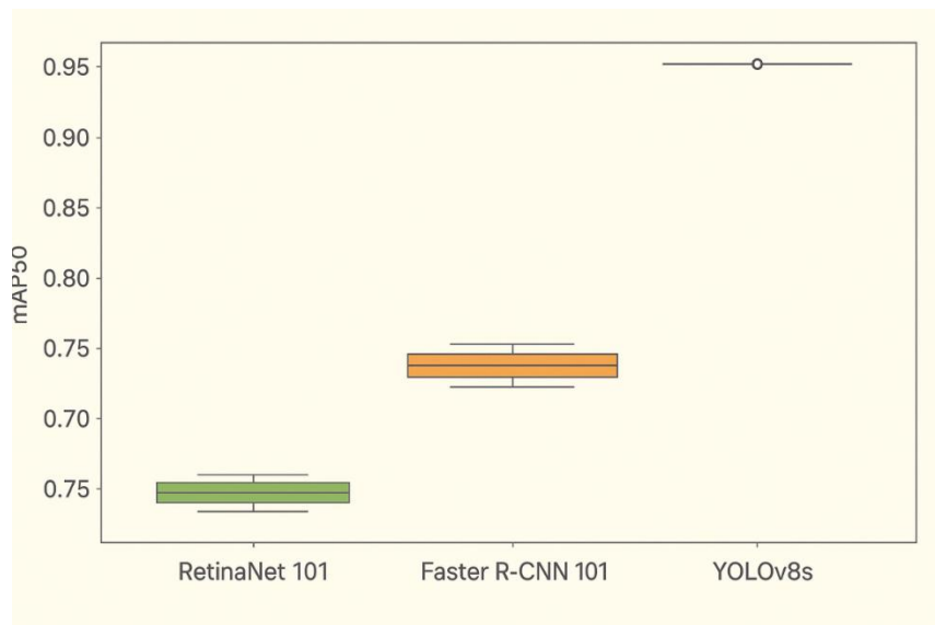
Figura 3: Diagrama de cajas de mean Average Precision (mAP 50 ) de los tres modelos
