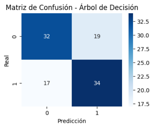
Figura 5. Matriz de confusión del modelo Árbol de Decisión
