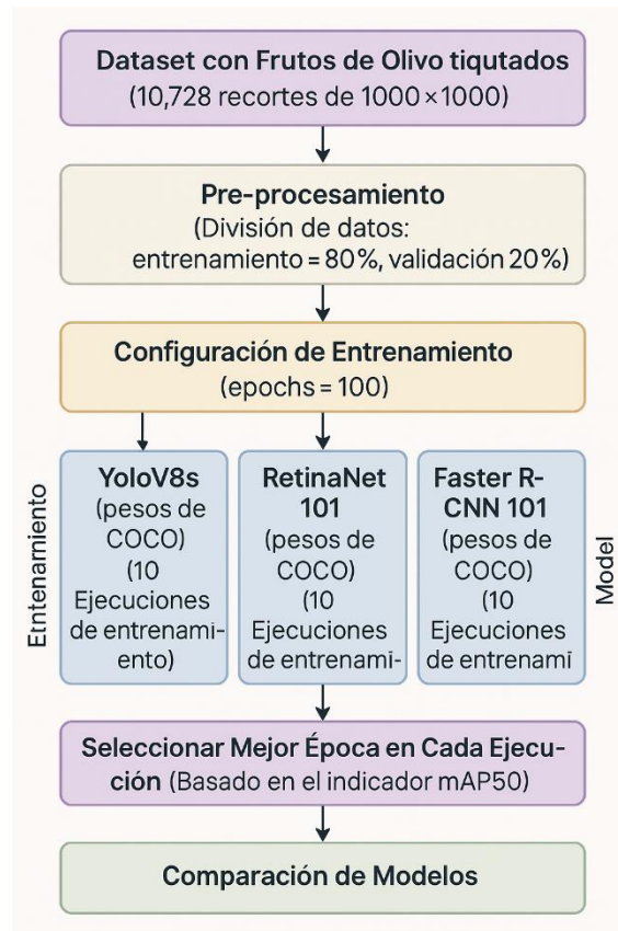
Figura 1. Flujo de trabajo y entrenamiento
