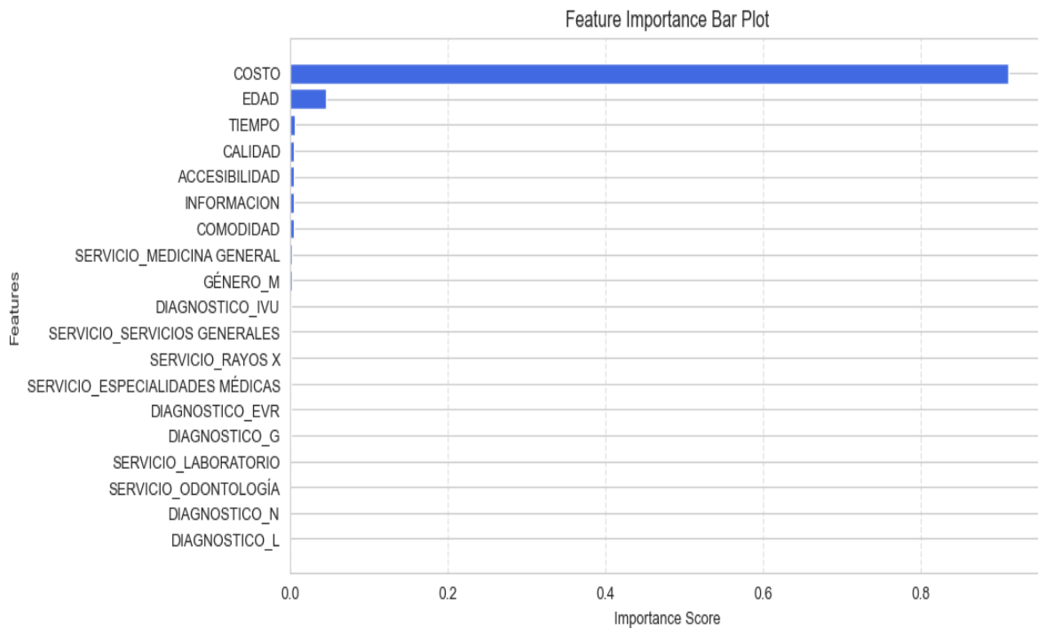
Figura 7. Importancia de las Variables en la Predicción del Beneficio Neto
