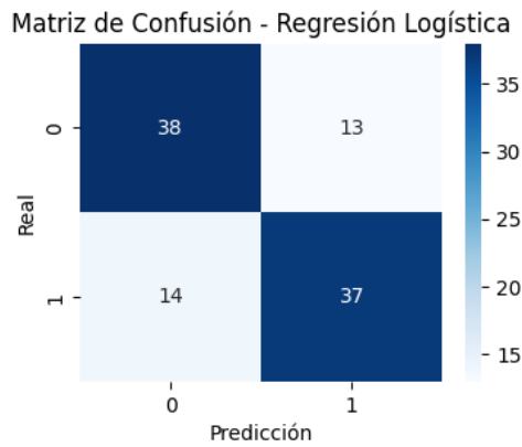
Figura 4. Matriz de confusión del modelo Regresión Logística
