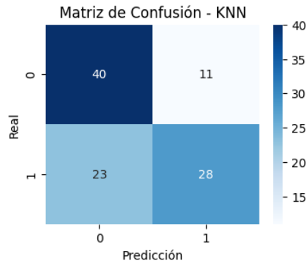
Figura 1. Matriz de confusión del modelo KNN
