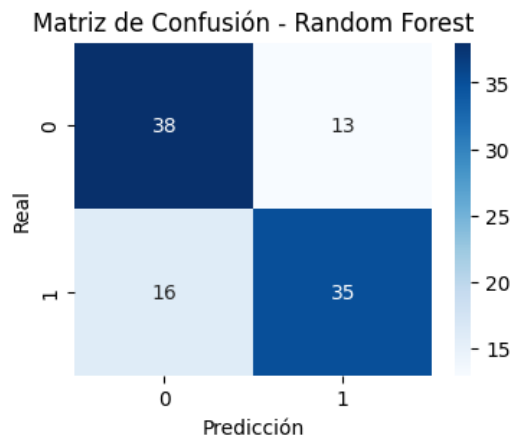
Figura 2. Matriz de confusión del modelo Random Forest
